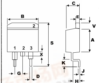
TO-263 (D2-PAK)
