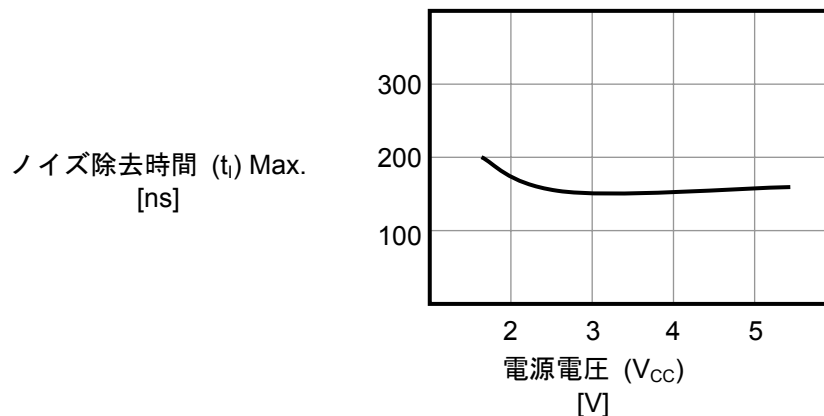
図 29 SDA 端子と SCL 端子ノイズ除去時間
