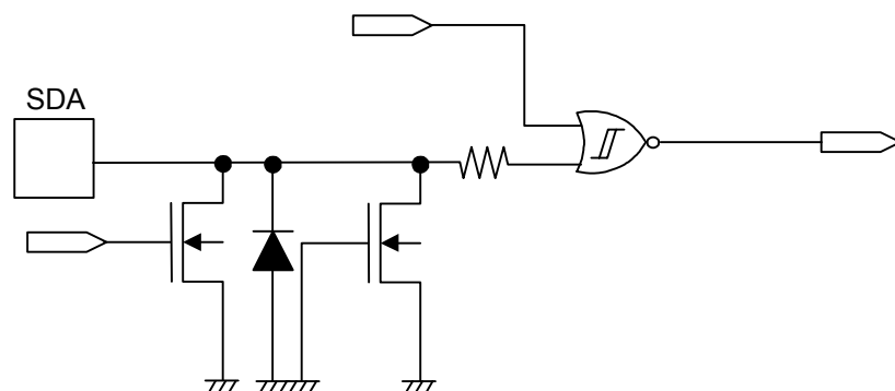
図 21 SDA 端子
