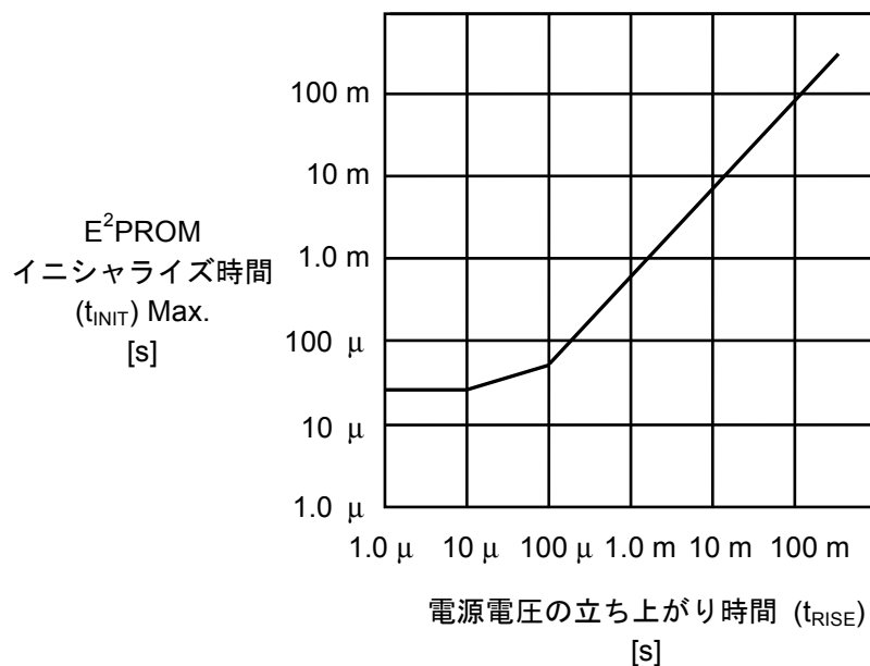
図 27 E 2 PROM のイニシャライズ時間
