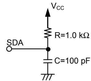
図5 出力負荷回路
