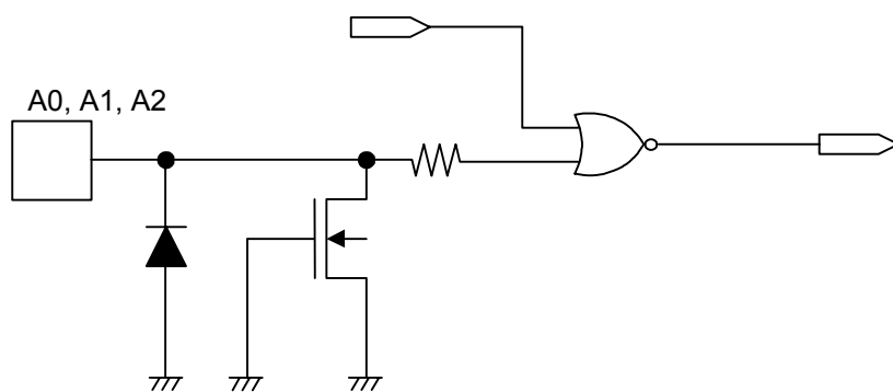
図 23 A0, A1, A2 端子
