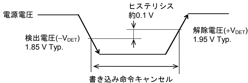
図19 低電源電圧時の動作
