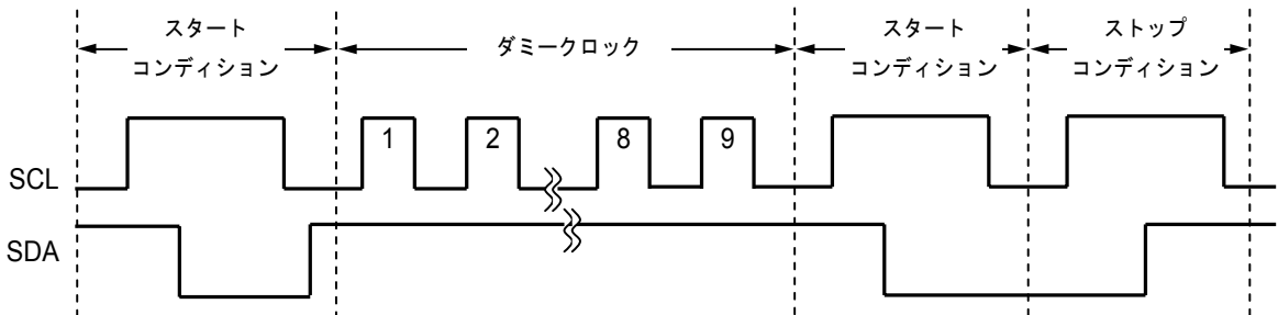
図24 E 2 PROMのリセット方法
