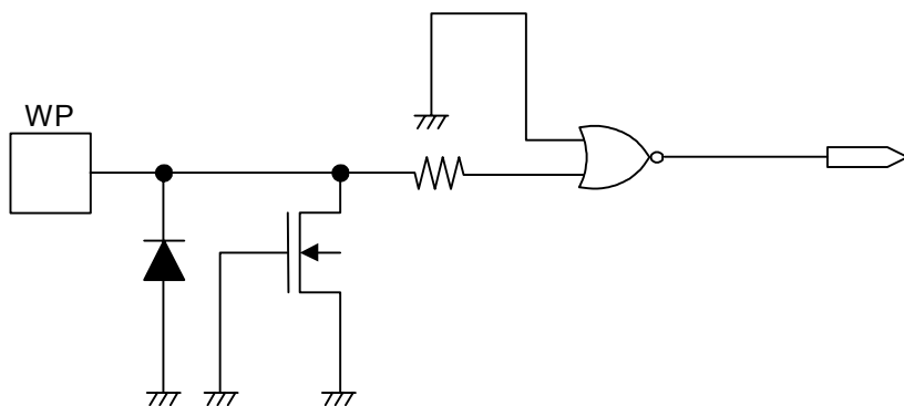
図 22 WP 端子
