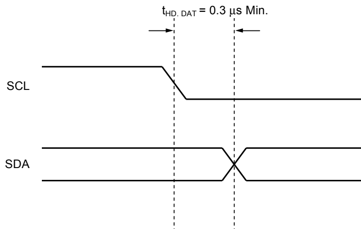
図 28 E 2 PROM のデータホールド時間
