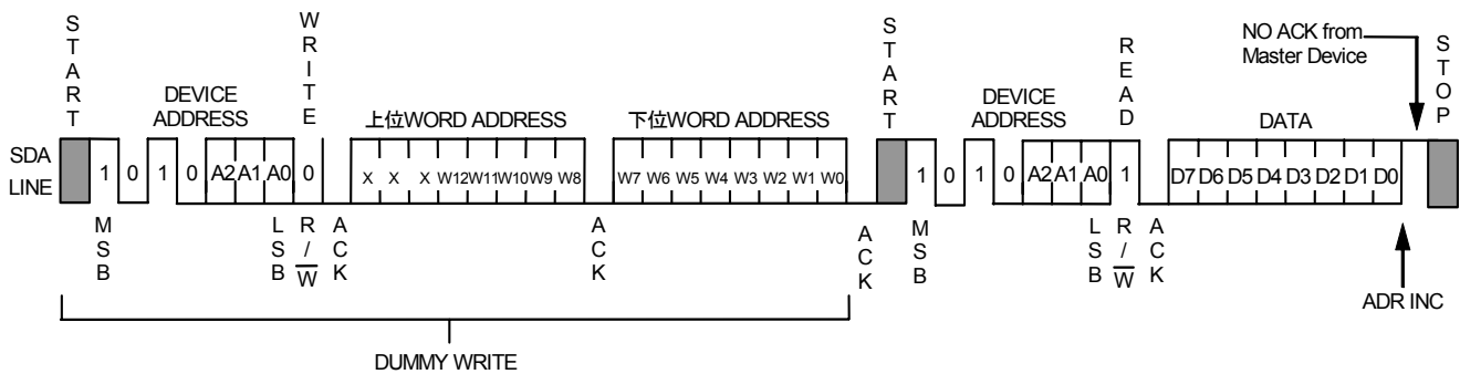
図15 ランダムリード
