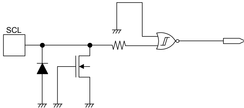
図 20 SCL 端子
