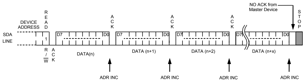
図16 シーケンシャルリード
