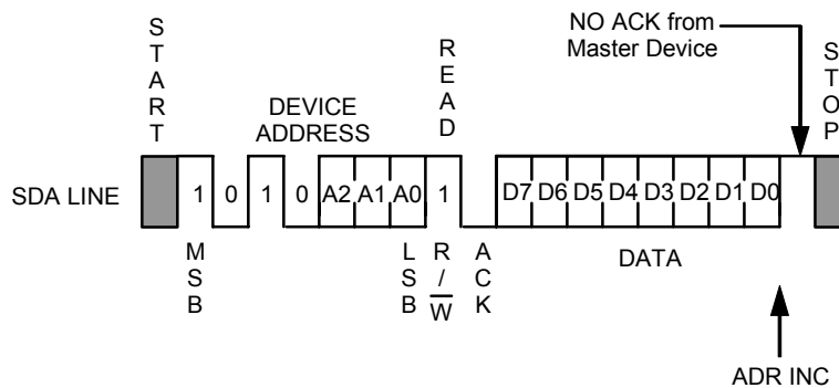
図14 カレントアドレスリード
