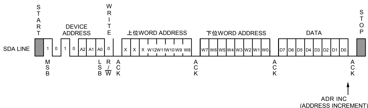
図12 バイトライト
