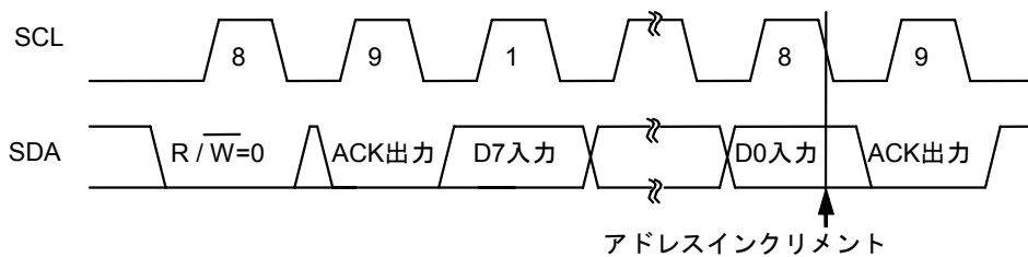
図18 書き込み動作時アドレスインクリメントタイミング
