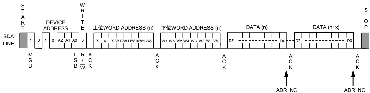
図13 ページライト
