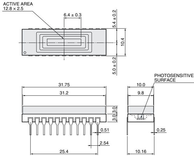
S3901-256F, S3904-512F
