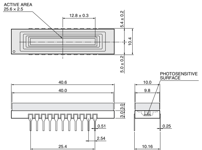
S3901-512F, S3904-1024F
