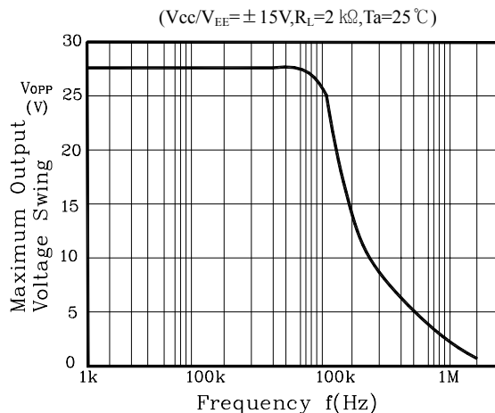
Fig. 2 V_{OP-P} - f
