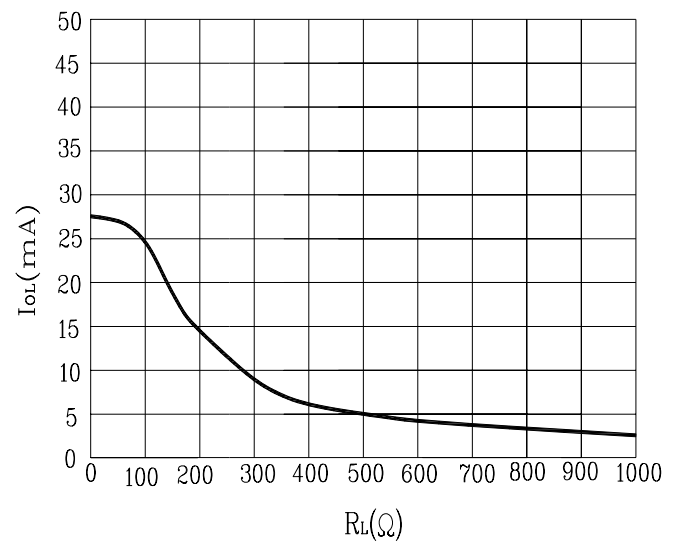
Fig. 4 I_{OL} - R_L
