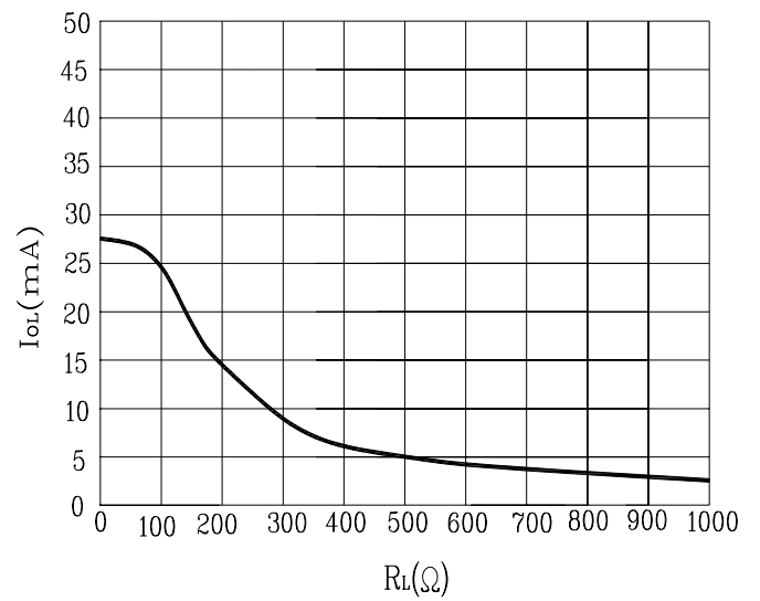
Fig. 4 I_{OL} - R_L
