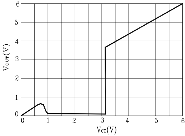
Fig. 1 V_{OUT} - V_{CC}
