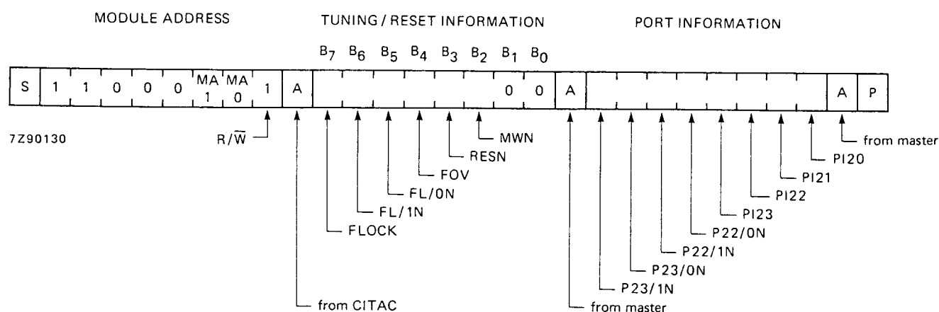
Fig. 6 Information byte format.
