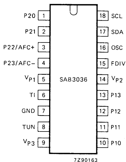
Fig. 2 Pinning diagram.
