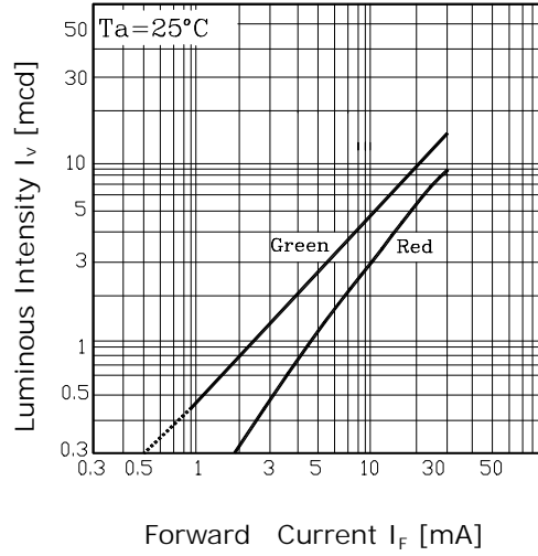
Fig. 2 I_V - I_F
