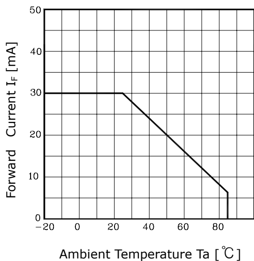
Fig. 3 I_F - T_a
