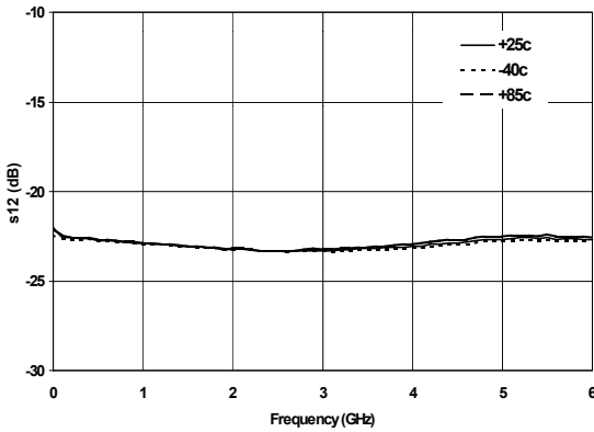
IS-95 @ 850MHz
