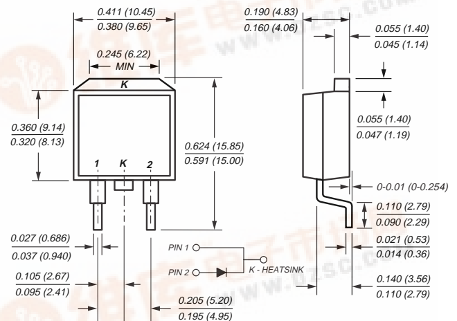
TO-263AB (SBLB10L25)
