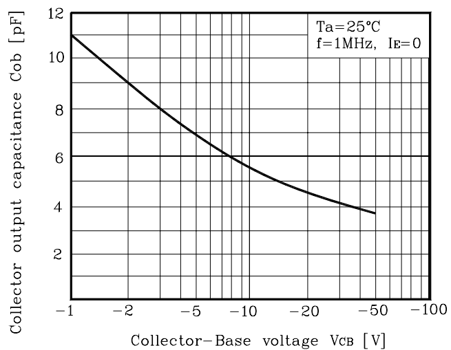
Fig. 4 C_{ob} - V_{CB}
