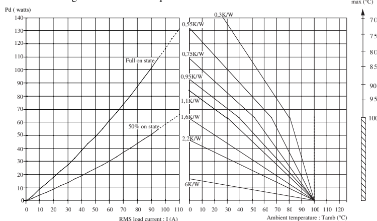
Fig. 2 Courbes thermiques / Thermal characteristics
