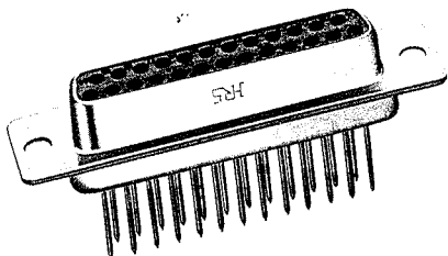
CL211-0324-2 SDBG-25S
