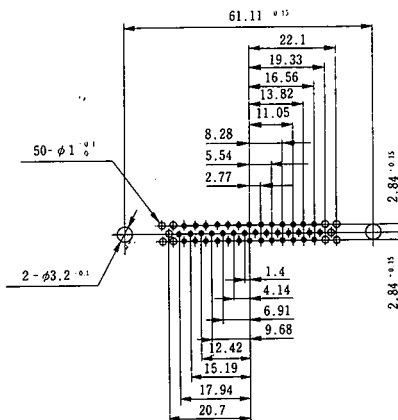
SDBB-25
