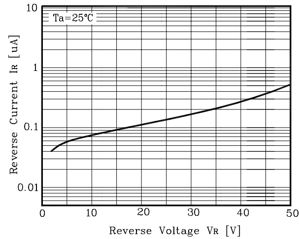
Fig. 2 I_R - V_R
