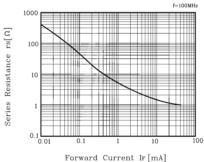
Fig. 2 r_s - I_F
