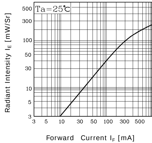
Fig. 2 I_E - I_F
