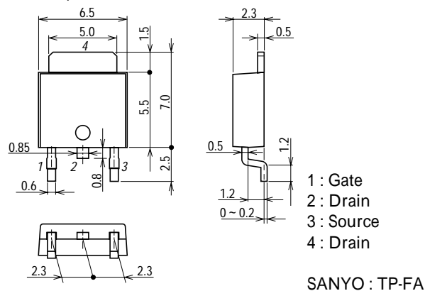
外形図 2092B
