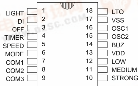
SM3502-A 18PIN
