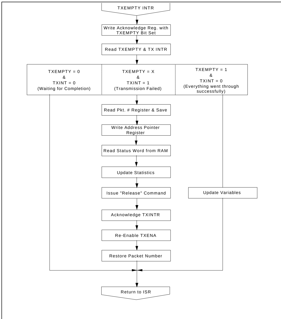
FIGURE 14 - TXEMPTY INTR
