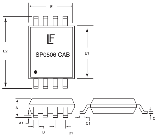
SP0506CAB - SOIC 8
