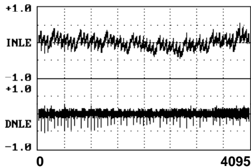
Vcc = 3.30V
