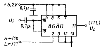
Bild 7: Typische Applikationsschaltung
