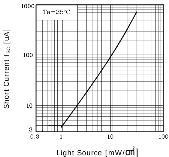
Fig. 1 I_{SC} - E_e
