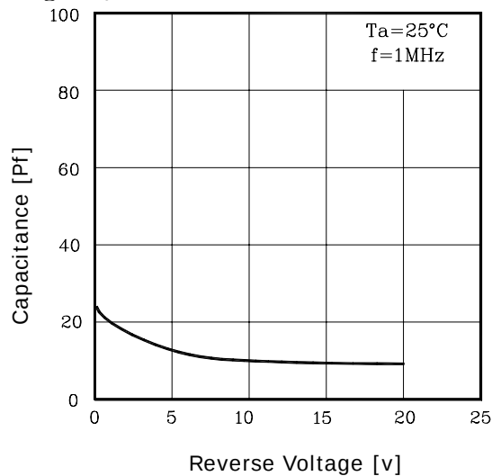
Fig. 3 C_t - V_R
