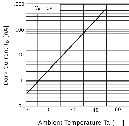
Fig. 2 I_D - T_a
