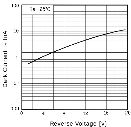
Fig.4 I_D - V_R
