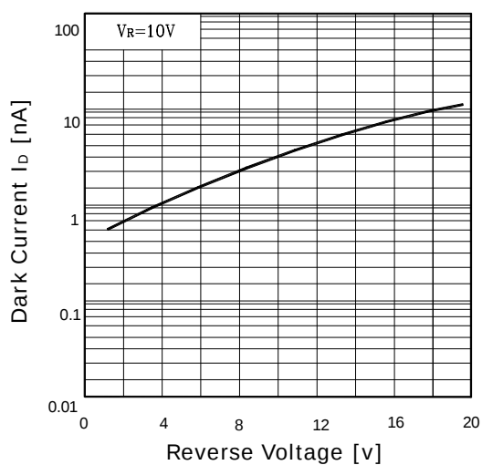
Fig. 4 I_D - V_R
