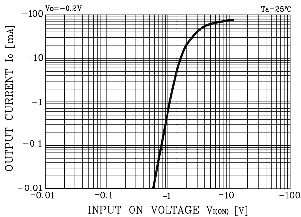
Fig. 3 G_1 - I_o
