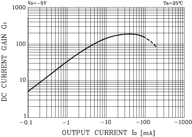
Fig. 3 G_1 - I_o
