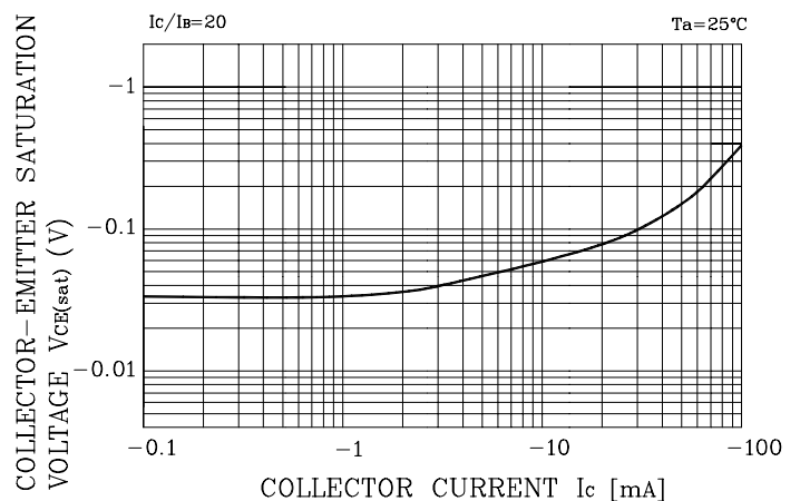
Fig. 2 V_{CE(SAT)} - I_C
