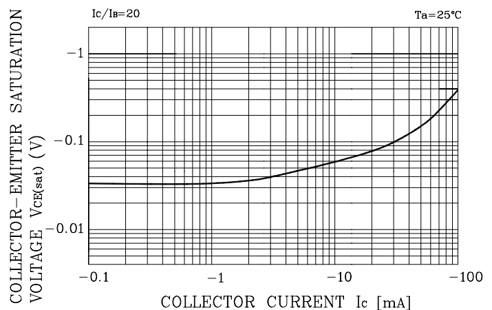
Fig. 2 V_{CE(SAT)} - I_C
