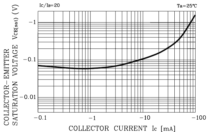
Fig. 2 V_{CE(SAT)} - I_C
