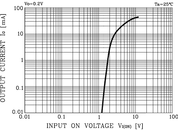
Fig. 3 G_1 - I_o
