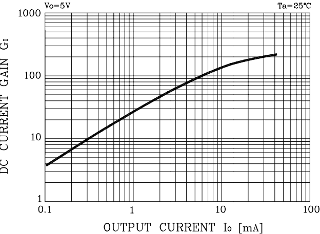
Fig. 3 G_1 - I_o
