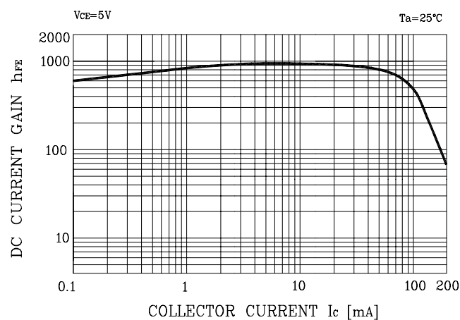
Fig. 1 h_{FE} - I_C
