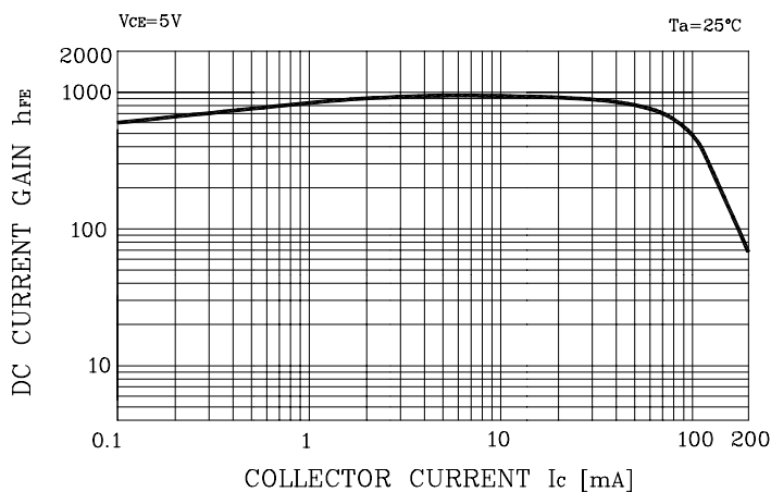
Fig. 1 h_{FE} - I_C
