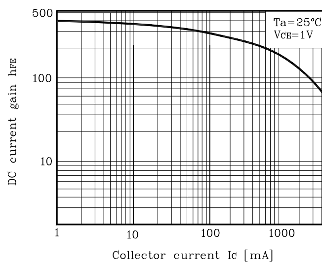
Fig. 4 h_{FE} - I_C
