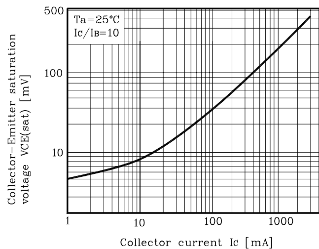
Fig. 2 V_{CE(sat)} - I_C
