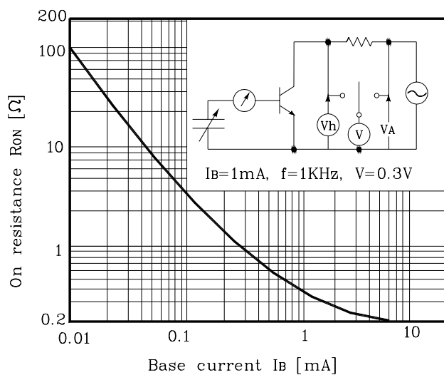
Fig. 5 R_{ON} - I_B
