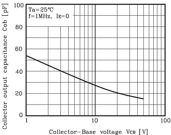
Fig. 5 C_{ob} - V_{CB}
