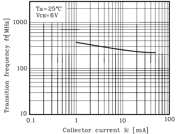
Fig. 4 f_T - I_C
