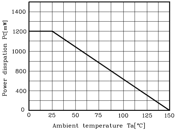
Fig. 1 P_c - T_a
