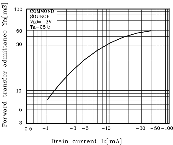
Fig5 |Y_{fs}| - I_D
