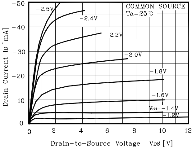
Fig1 I_D - V_{DS}
