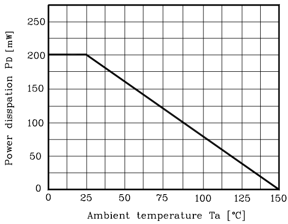
Fig9 Pd - Ta
