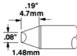
STTC-X14 Bevel 45° .08~ (2.03mm)
