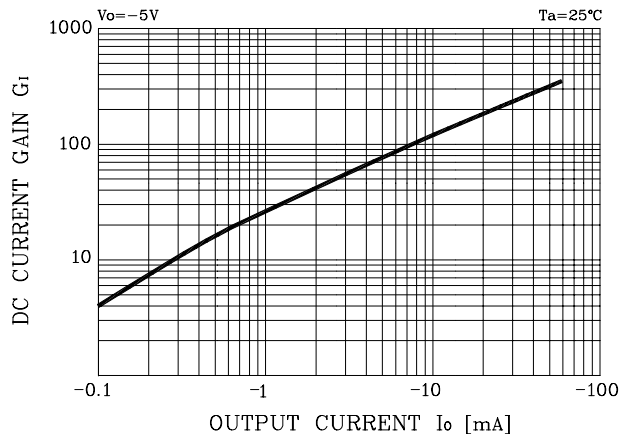
Fig. 3 G_I - I_O
