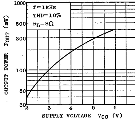
POUT - V_{CC}
