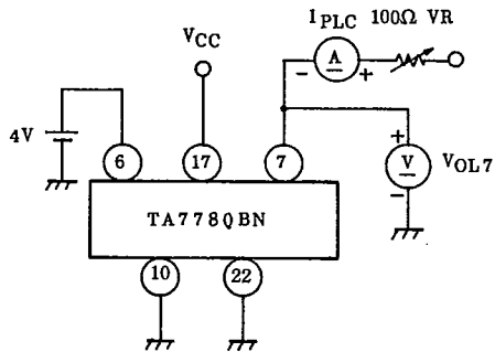
TEST CIRCUIT 7 : VOL7
