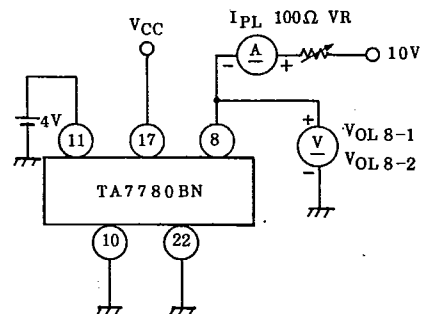
TEST CIRCUIT 6 : V_{OL8-1} , V_{OL8-2}
