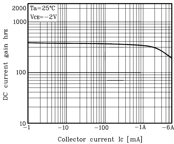
Fig. 3 h_{FE} - I_c
