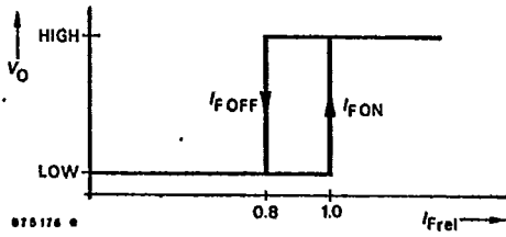
Fig. 3 Hysteresis
