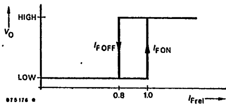
Fig. 3 Hysteresis
