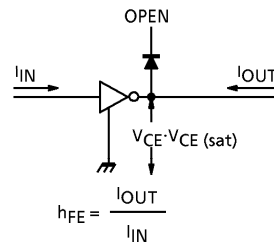
2. V CE (sat) , h FE
