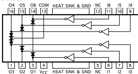
TD62309F
