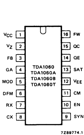
Fig. 2 Pinning diagram.
