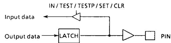
Figure1-2. Port P3
