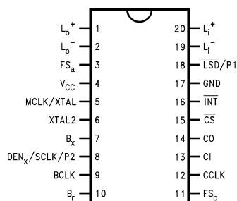
TP3420A SID
