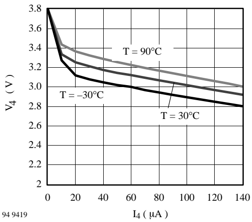
V_4 (Pin 4) versus I_4
